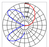
Max Candela linea 3ft 132.5° vertical = 865 180° horizontal = 865
