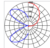
Max Candela linea mini 130° vertical = 178 180° horizontal = 178
